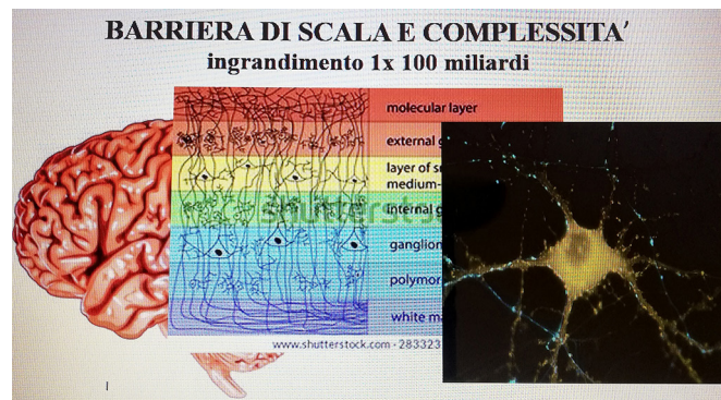
Figura 1: Barriera di scala e complessità, 100 miliardi di ingrandimenti scalari necessari all'osservazione del singolo neurone corticale a partire dalla superficie cerebrale.
